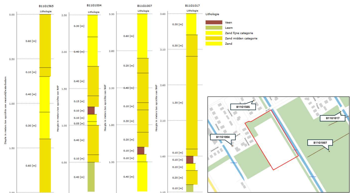
Figuur 2-4: Boormonsterprofielen en locaties van grondboringen met plangebied (bron: DINOlaket).
