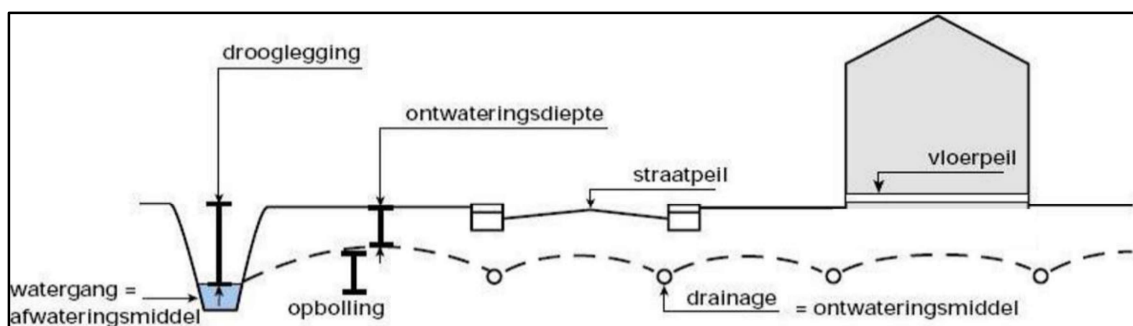
Figuur 4-4: Schematische weergave ontwateringsdiepte.
