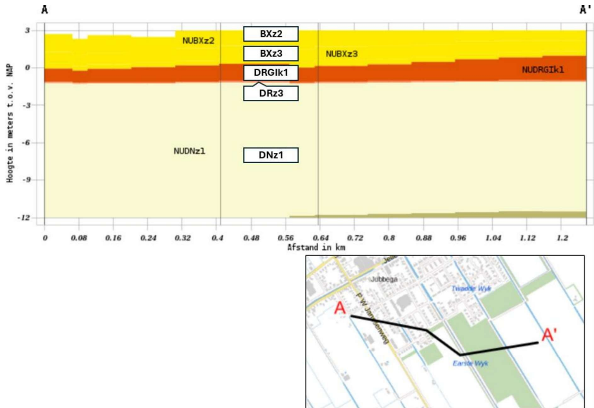
Figuur 2-3: Geohydrologisch profiel op basis van REGIS II v2.2.3 (bron: DINOlaket).
