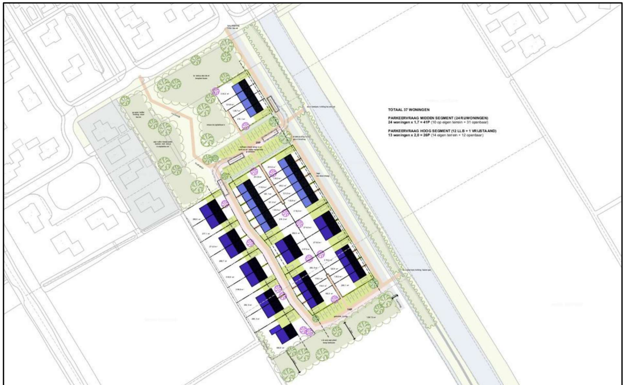
Figuur 1-1: Weergave van het planvoornemen, variant 1 (links) en variant 2 (rechts) (bron: VMEZ Architecten).
