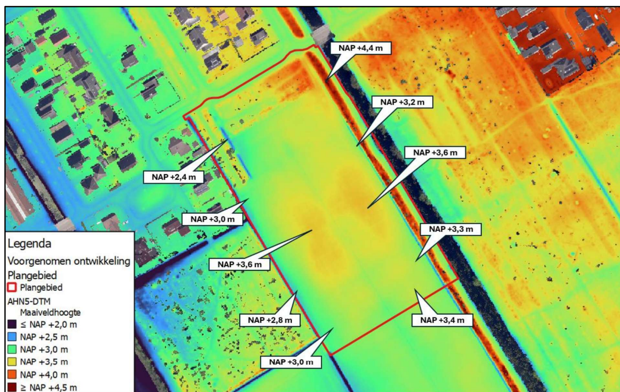
Figuur 2-2: Maaiveldhoogten plangebied (bron: AHN5-DTM).
