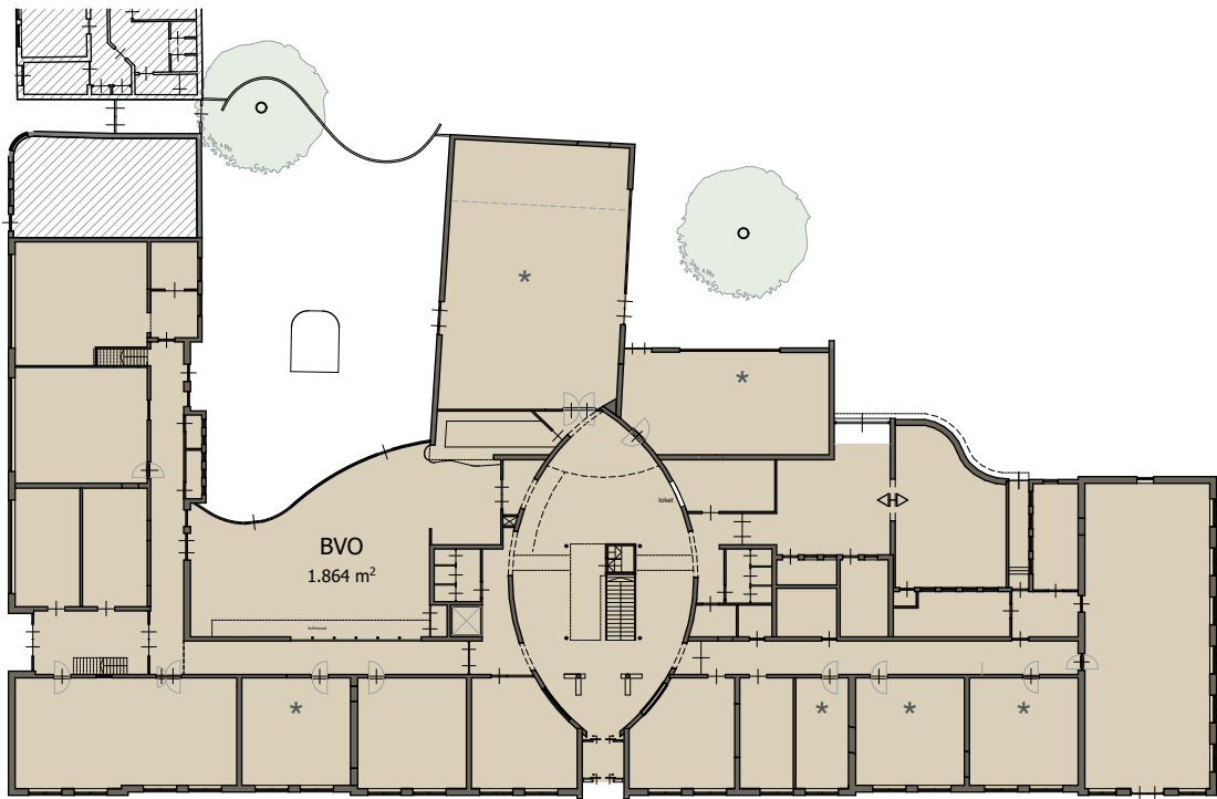
begane grond
